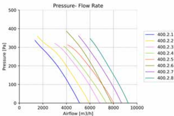
Ø400 / 3-4-5 Blade
